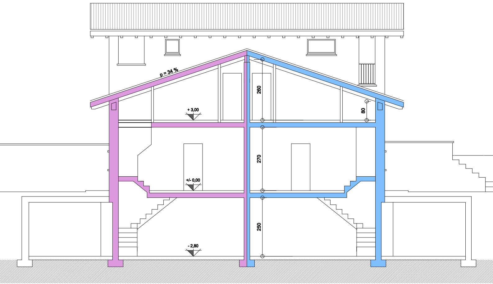
SEZIONE A - A
